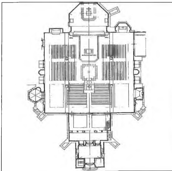
St. Petrus - Leiden (III) - az átalakítás után (1990)
